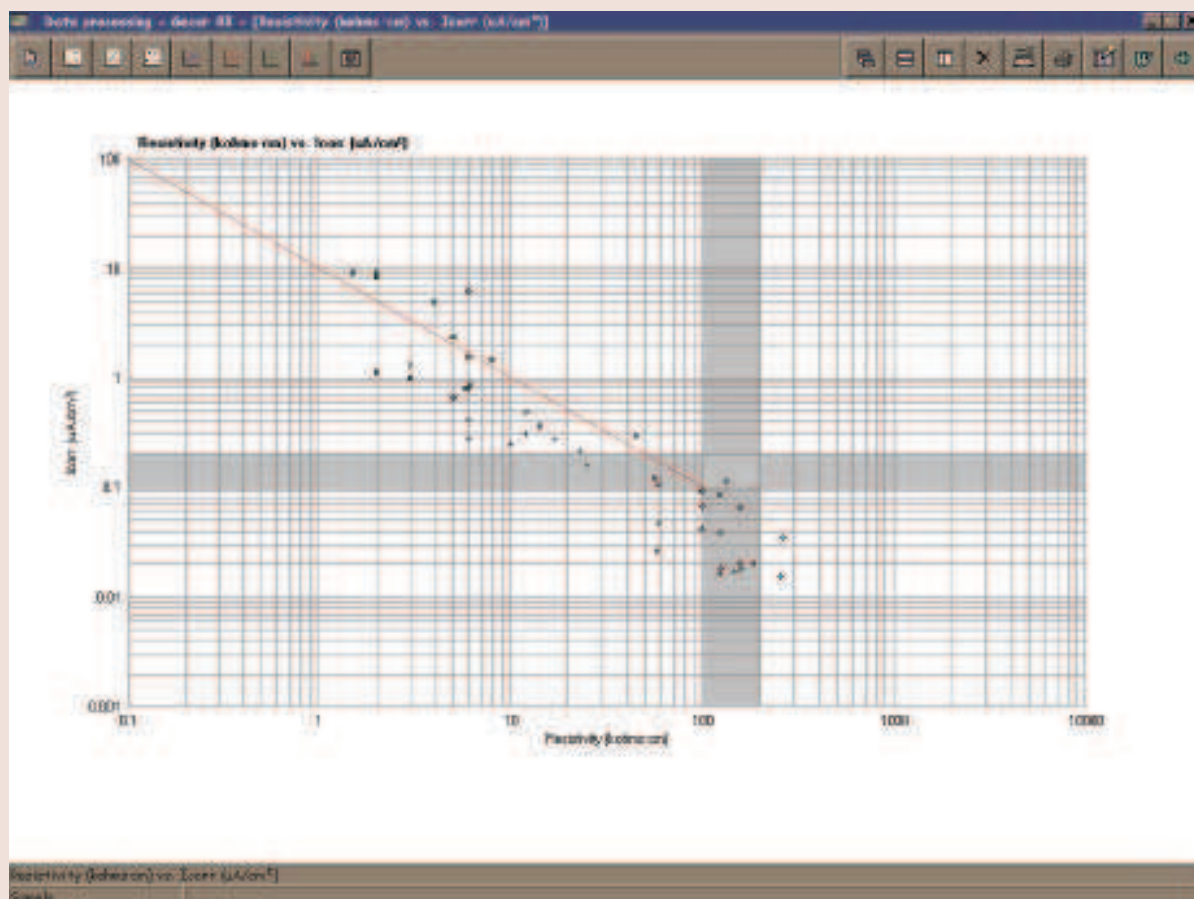
Resistividad Contra Densidad Actual de Corrosión
